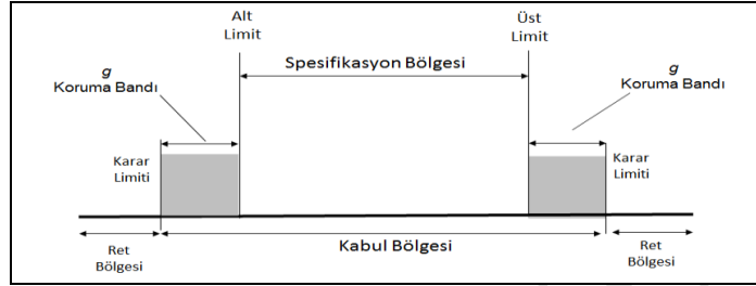
Şekil VII: Alt ve Üst Limite Dayanan Kabul ve Ret Bölgesi
